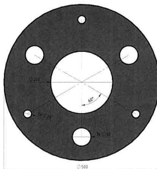
Blacha czołowa dolna (poz. 3) \phi 500 \times 5\text{mm}
