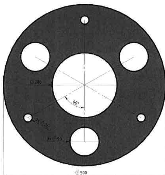
Blacha czołowa górna (poz. 2) \phi 500 \times 5\text{mm}
