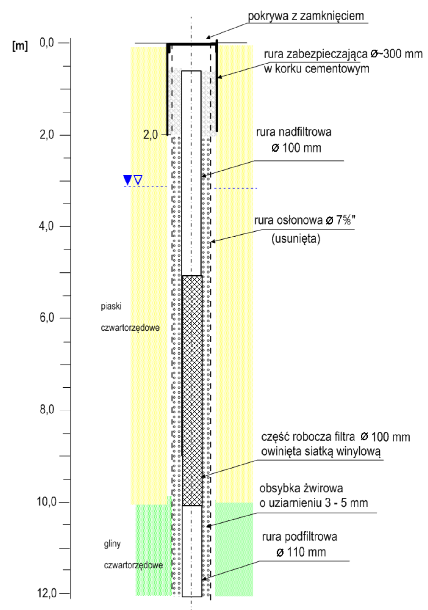
Profil geologiczno-techniczny otworu do badań hydrogeologicznych (P)
